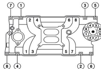
ORDRE D'ALLUMAGE 1-8-4-3-6-5-7-2
