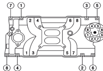
ORDEN DE EXPLOSIÓN 1-8-4-3-6-5-7-7
