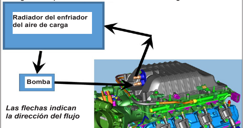
Diagrama esquemático de enfriador de aire de carga estilo Camaro
