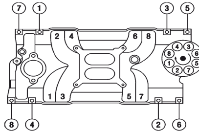
ORDRE D'ALLUMAGE 1-8-4-3-6-5-7-2
