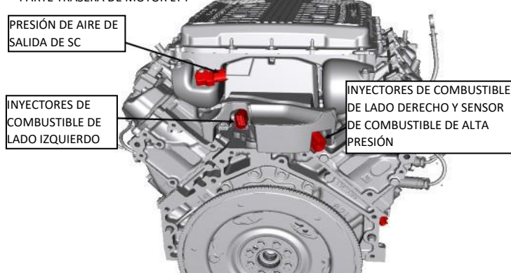
PARTE TRASERA DE MOTOR LT4
