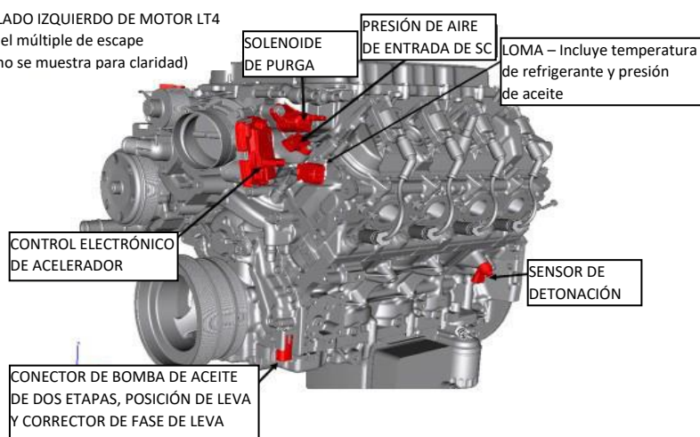
LADO IZQUIERDO DE MOTOR LT4
