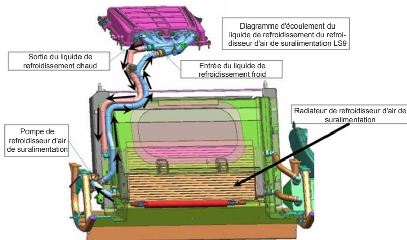
Montage typique du refroidisseur d'air de suralimentation
