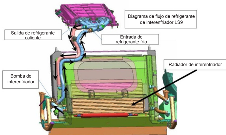
Configuración de enfriador de aire de carga típico
