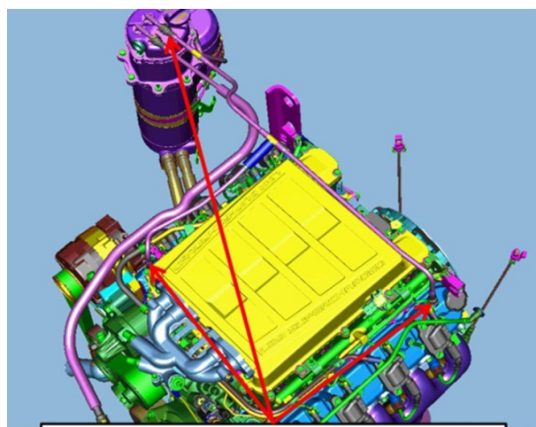
Ventilación positiva de cárter (PCV): Conecta las cubiertas del tanque de sumidero seco al balancín
